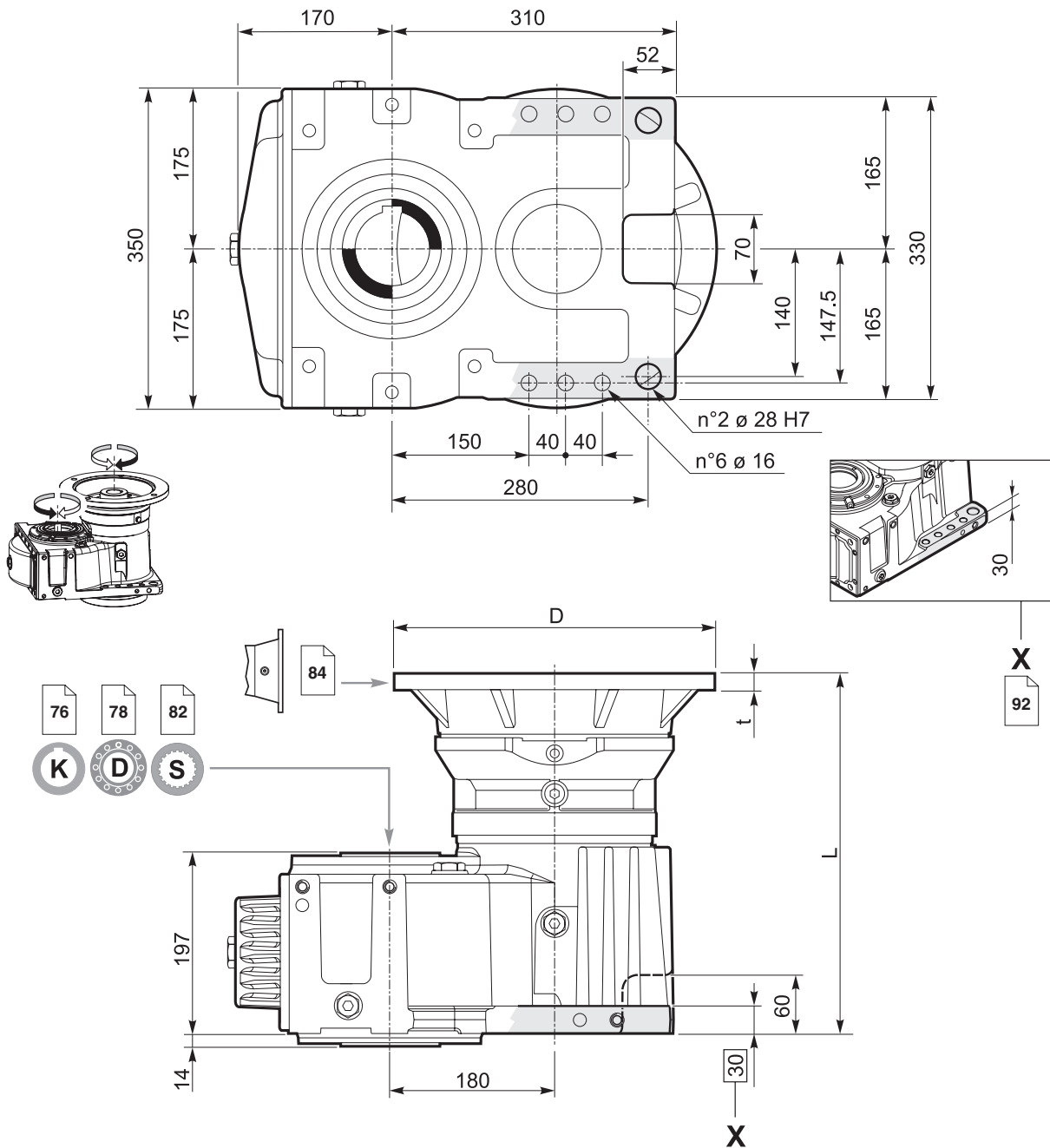
Motorlanterne IEC / IEC Adaptor / Predisposizioni IEC / Prédiposition IEC / Preparado para el motor IEC / Adaptador IEC
