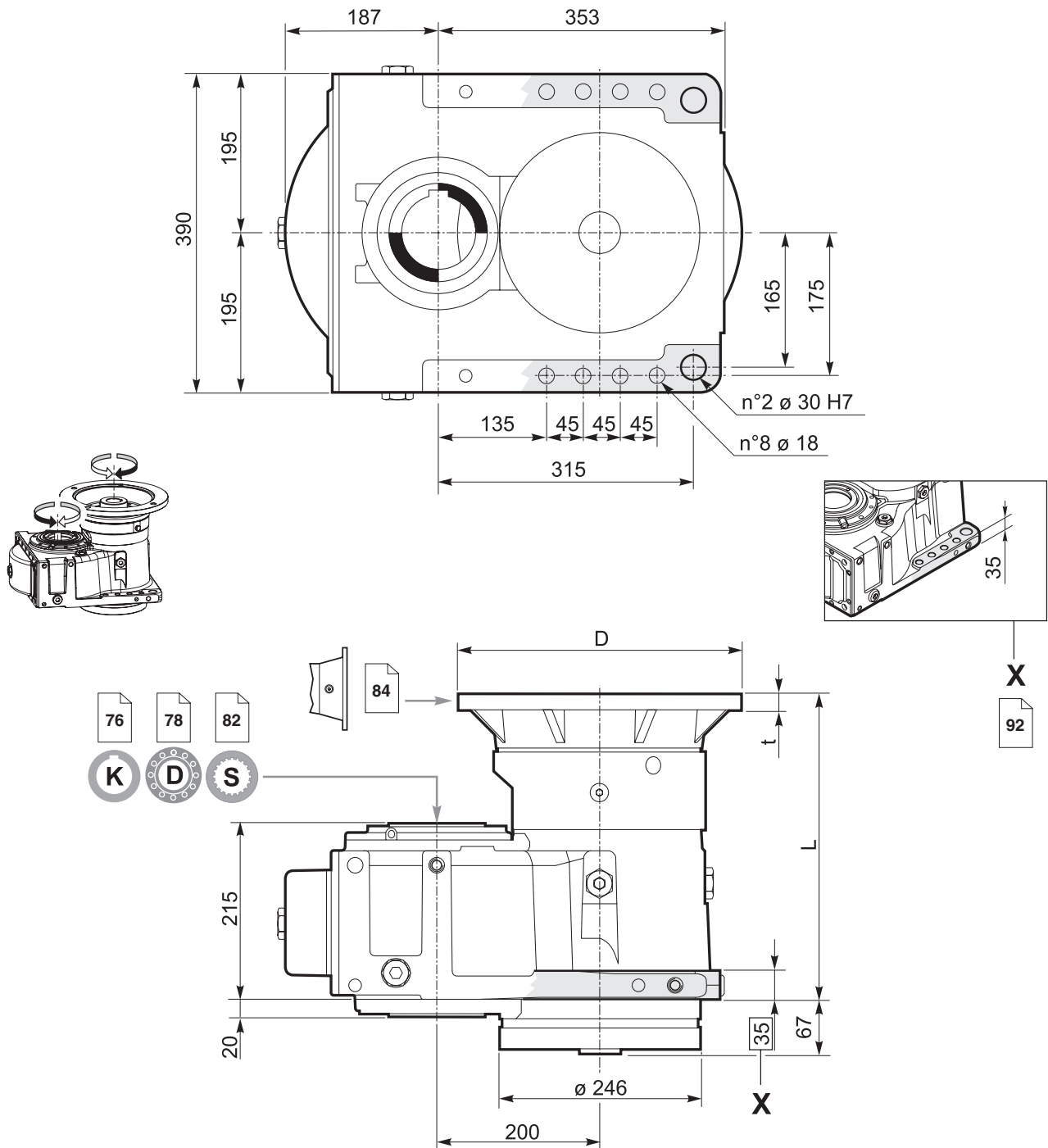
Motorlaterne IEC / IEC Adaptor / Predisposizioni IEC / Prédisposition IEC / Preparado para el motor IEC / Adaptador IEC
