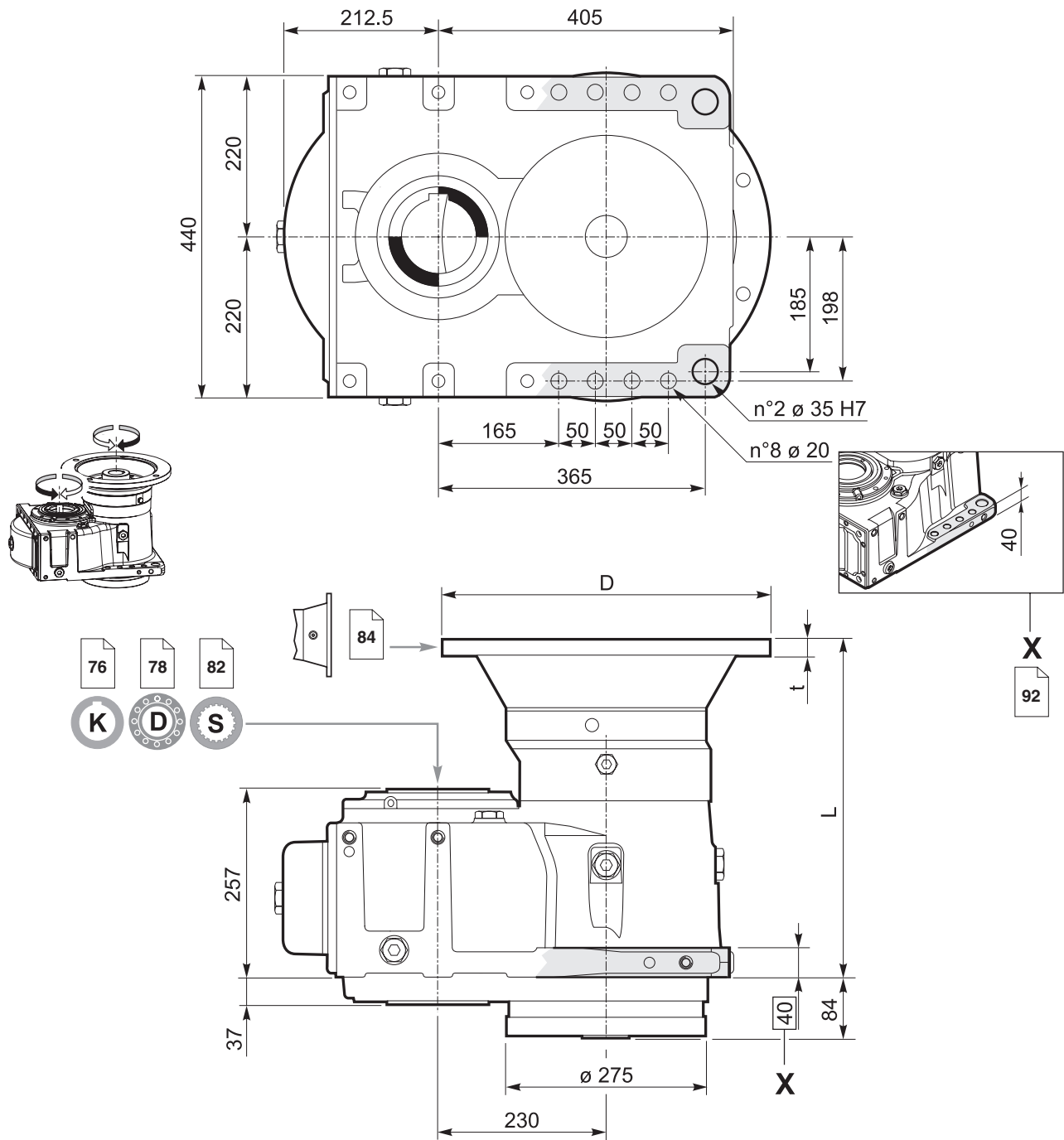
Motorlaterne IEC / IEC Adaptor / Predisposizioni IEC / Pr disposition IEC / Preparado para el motor IEC / Adaptador IEC
